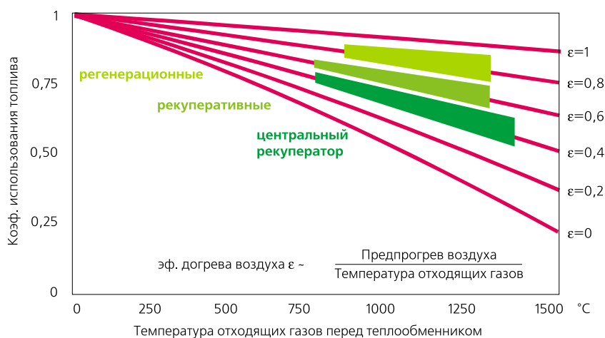
Рис. 1. КИТ как зависимость температуры отходящих газов и эффективности догрева воздуха
