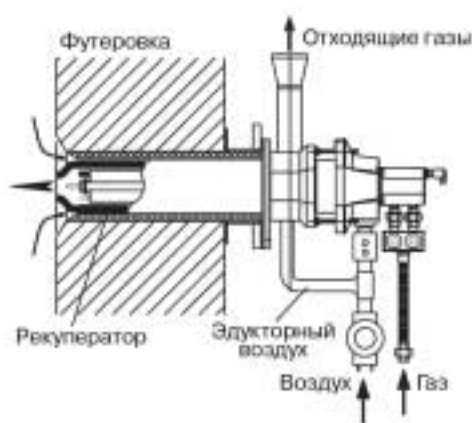
Рис. 2. REKUMAT MSJ 200 для прямого нагрева
